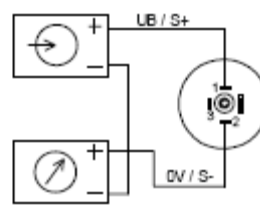
výstup 2-vodič s konektorem 803 C
