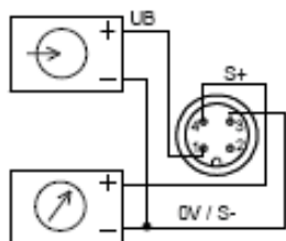
výstup 3-vodič s konektorem M12x1,5
