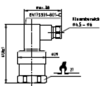
S konektorem typ 803 C
