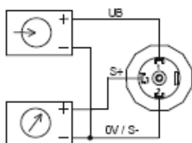
výstup 3-vodič s konektorem 803 A
