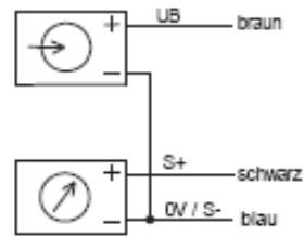
výstup 3-vodič s kabelem
