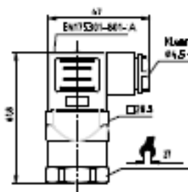
S konektorem typ 803 A
