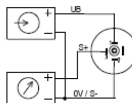
výstup 3-vodič s konektorem 803 C
