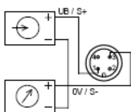
výstup 2-vodič s konektorem M12x1,5
