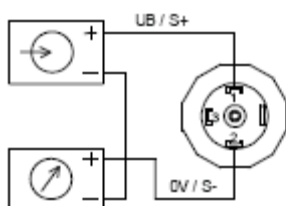
výstup 2-vodič s konektorem 803 A
