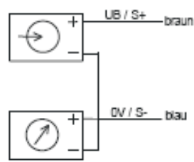
výstup 2-vodič s kabelem
